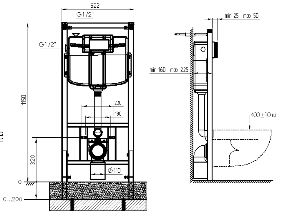
Рис.2 ОСНОВНЫЕ РАЗМЕРЫ:
